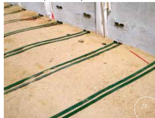
Armaduras EcoStrap™ HA® en Chessy.
